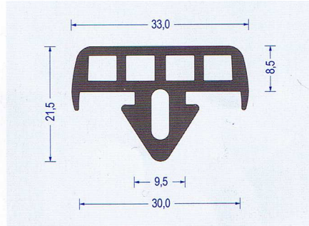
Art.-Nr. 2330002 EPDM 70 °Shore A schwarz VE : 25 m Bund
