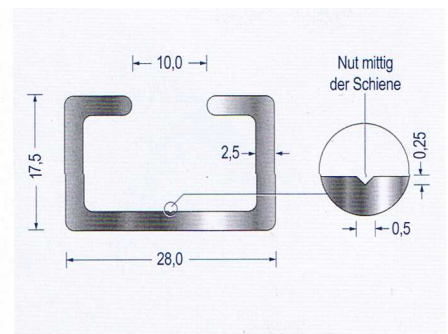
Art.-Nr. 2330008 Halteleiste für Polsterprofil ( nicht geeignet für Profil Art.-Nr. 2330006) Aluminium blank VE : Länge á 5 m Bund . Mindestmenge 10 m
