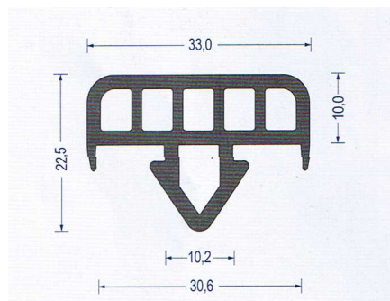
Art.-Nr. 2330007 EPDM 60 °Shore A schwarz VE : 25 m Bund
