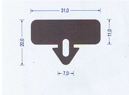
Art.-Nr. 2330001 EPDM 65 °Shore A schwarz VE : 25 m Bund
