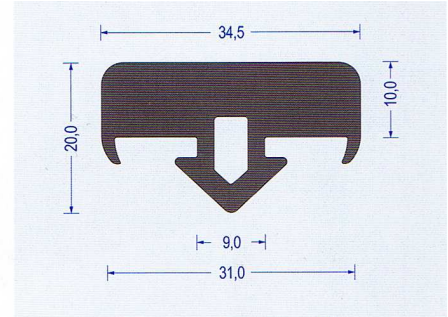
Art.-Nr. 2330003 EPDM 70 °Shore A schwarz VE : 25 m Bund
