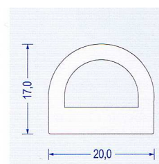
Art.-Nr. 2740009 60° Shore A · transluzent VE : 25 m Bund
