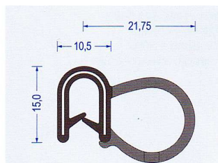
Art.-Nr. 2830016 CR schwarz Klemmber. 1-3,5 mm VE : 25 m Bund Br* a200/b80/c200/d200
