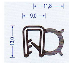
Art.-Nr. 2830005 NBR schwarz Klemmber. 2 mm VE : 50 m Bund Br* a50/b20/c120/d40
