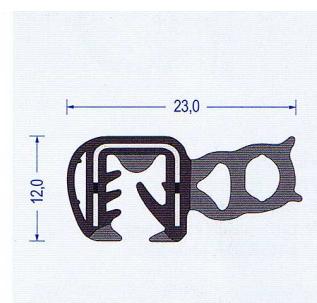
Art.-Nr. 2830034 EPDM schwarz Klemmber. 4-6 mm VE : 50 m Bund
