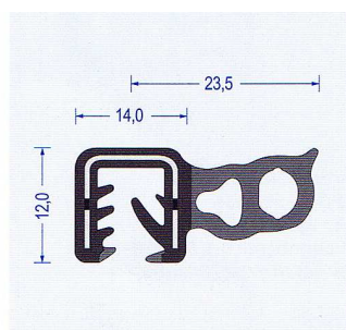
Art.-Nr. 2830033 EPDM schwarz Klemmber. 4-6 mm VE : 50 m Bund
