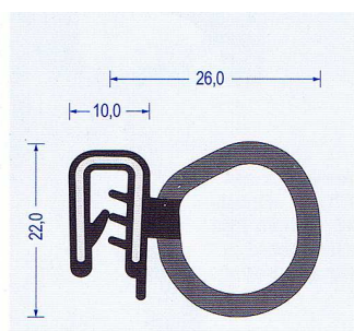
Art.-Nr. 2830032 EPDM schwarz Klemmber. 1-3,5 mm VE : 50 m Bund
